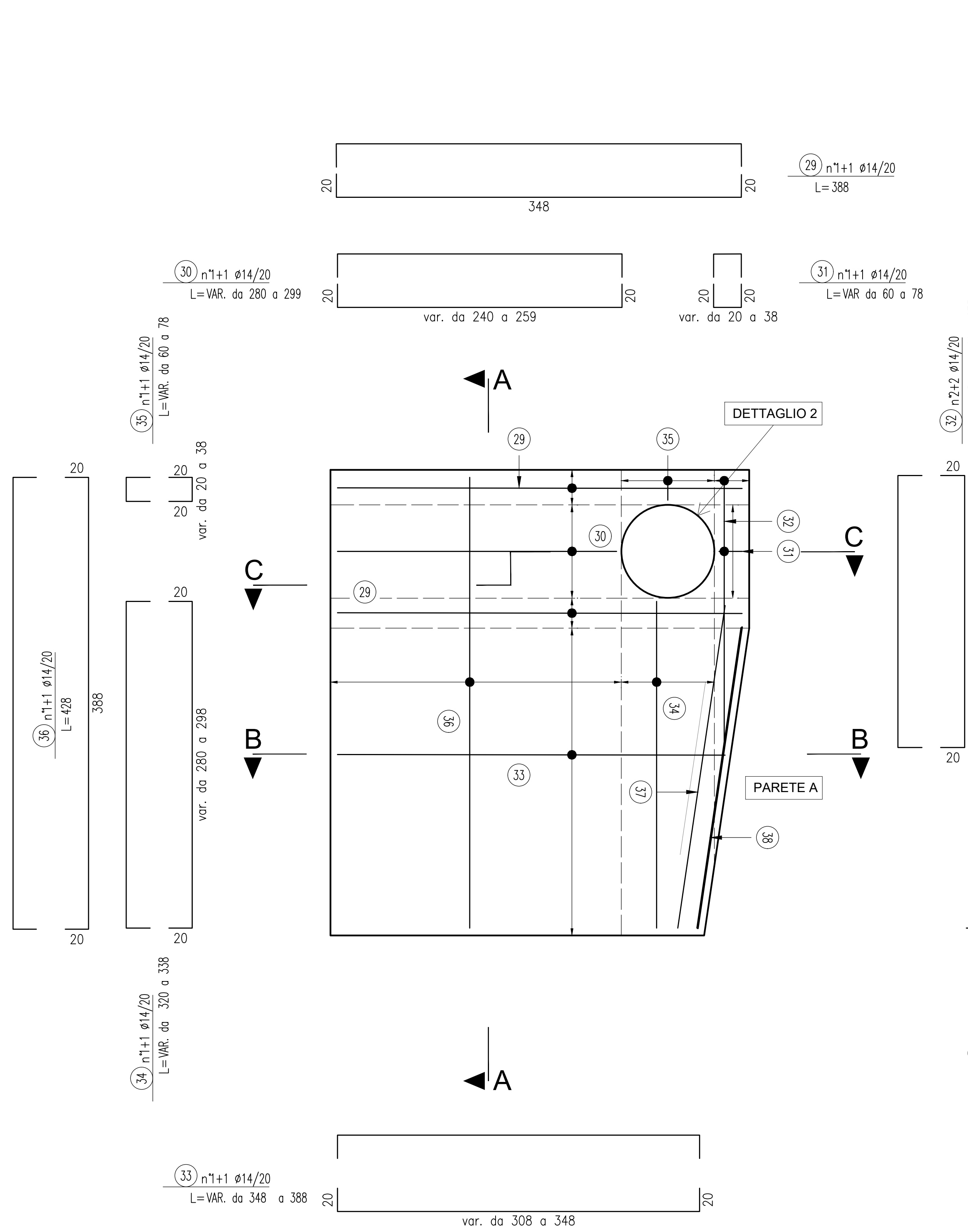
PIANTA COPERTURA (scala 1:25)
