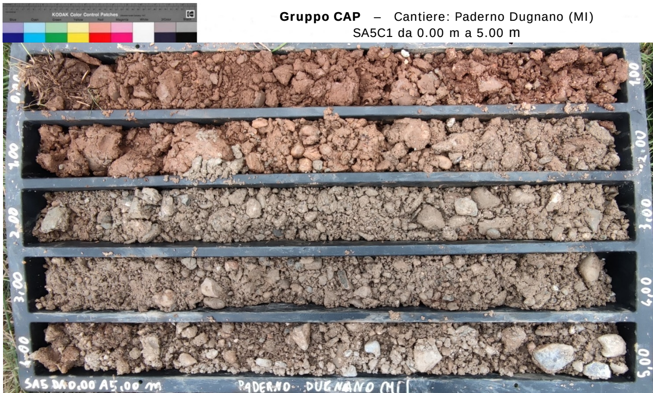
Foto 13. Sondaggio SA5 da 0.00 m a 5.00 m.
