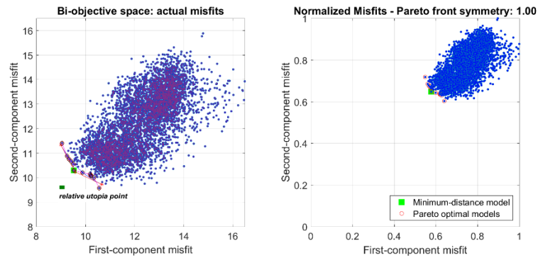
Figura 41. Diagramma distribuzione pareto ed errori attuale
