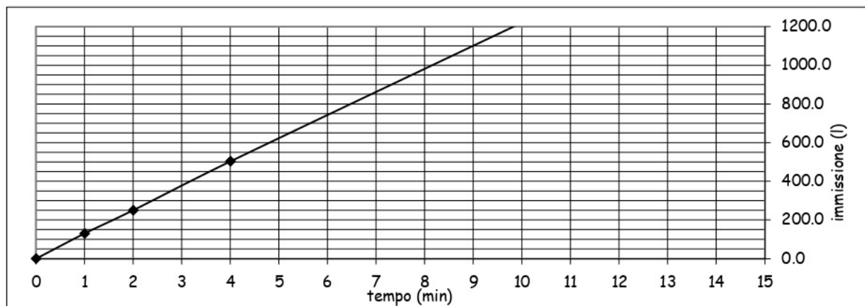
Figura 24. Risultati prova di permeabilità S2 K2.
