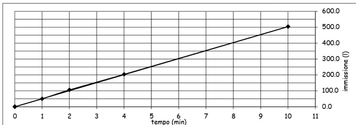
Figura 27. Risultati prova di permeabilità S3 K2.
