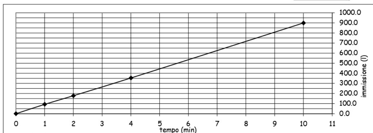
Figura 23. Risultati prova di permeabilità S2 K1.
