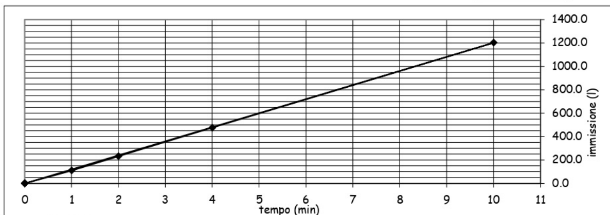
Figura 22. Risultati prova di permeabilità S1 K1.
