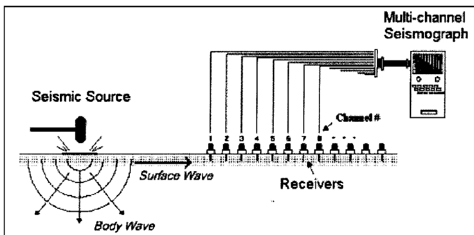
Figura 33. Schema stendimento sismico MASW
