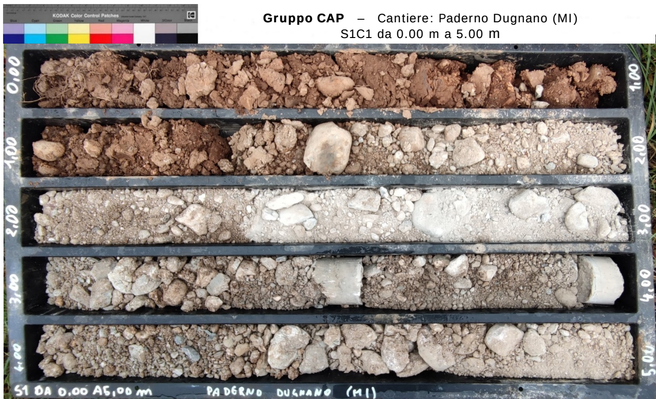
Foto 1. Sondaggio S1 da 0.00 m a 5.00 m.
