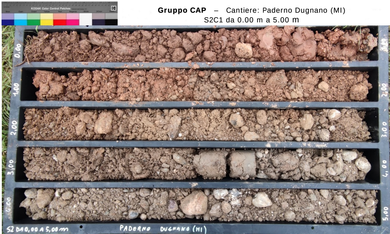
Foto 2. Sondaggio S2 da 0.00 m a 5.00 m.
