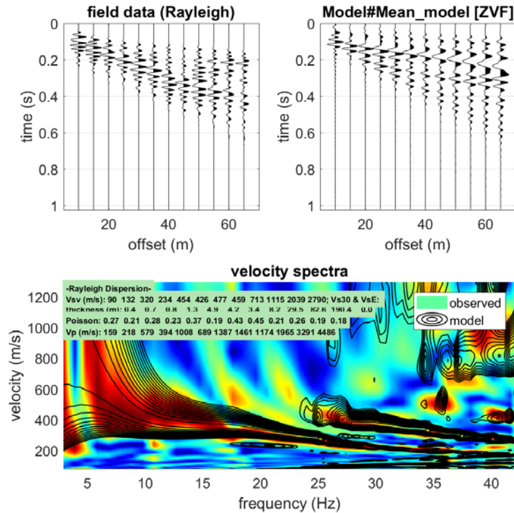
Figura 39. Modello distanza minima in full velocity spectral per le onde di Rayleigh
