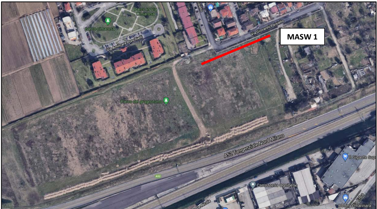
Figura 34. Ubicazione indagini MASW
