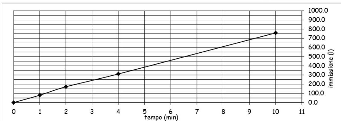
Figura 25. Risultati prova di permeabilità S2 K3.
