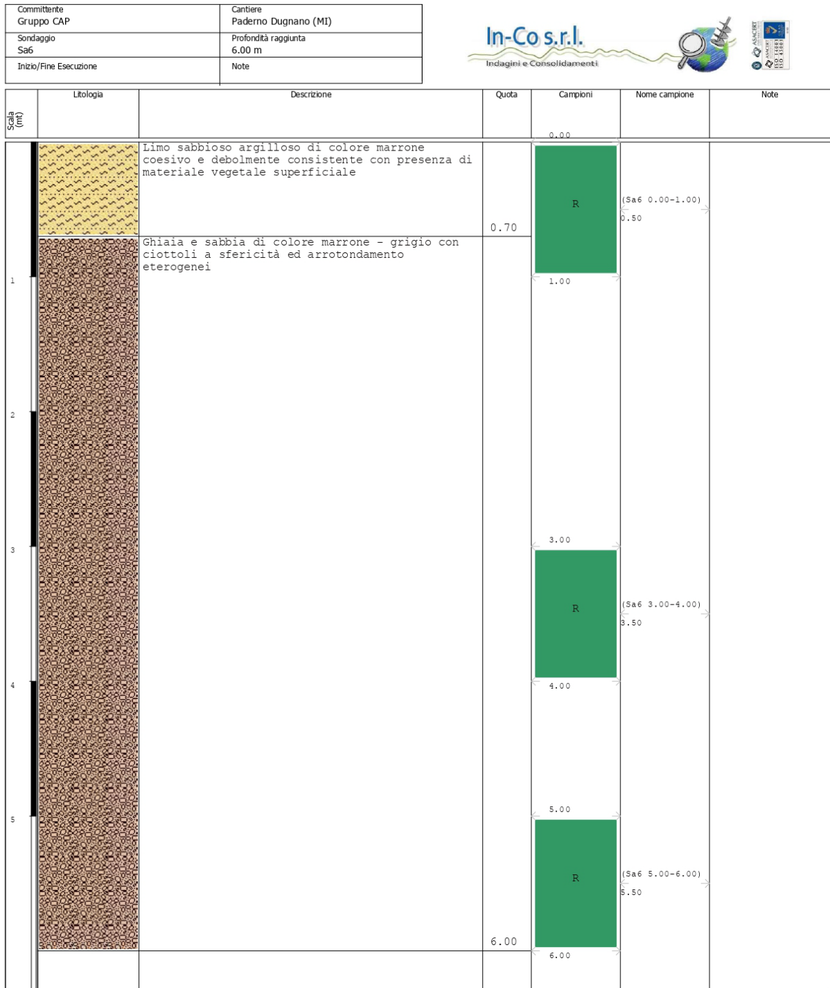
Figura 18. Stratigrafia del sondaggio Sa6.
