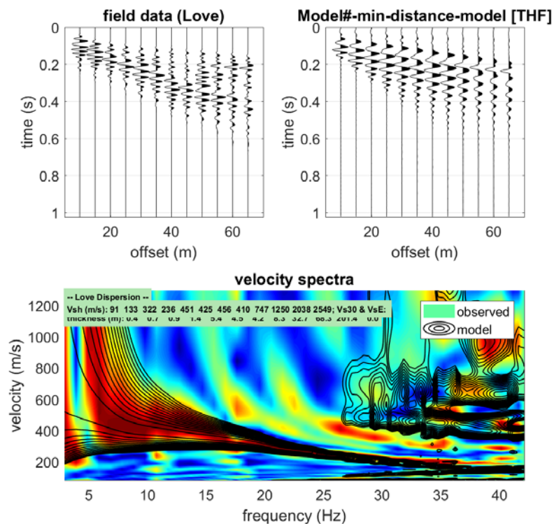
Figura 40. Modello distanza minima in full velocity spectral per le onde di Love
