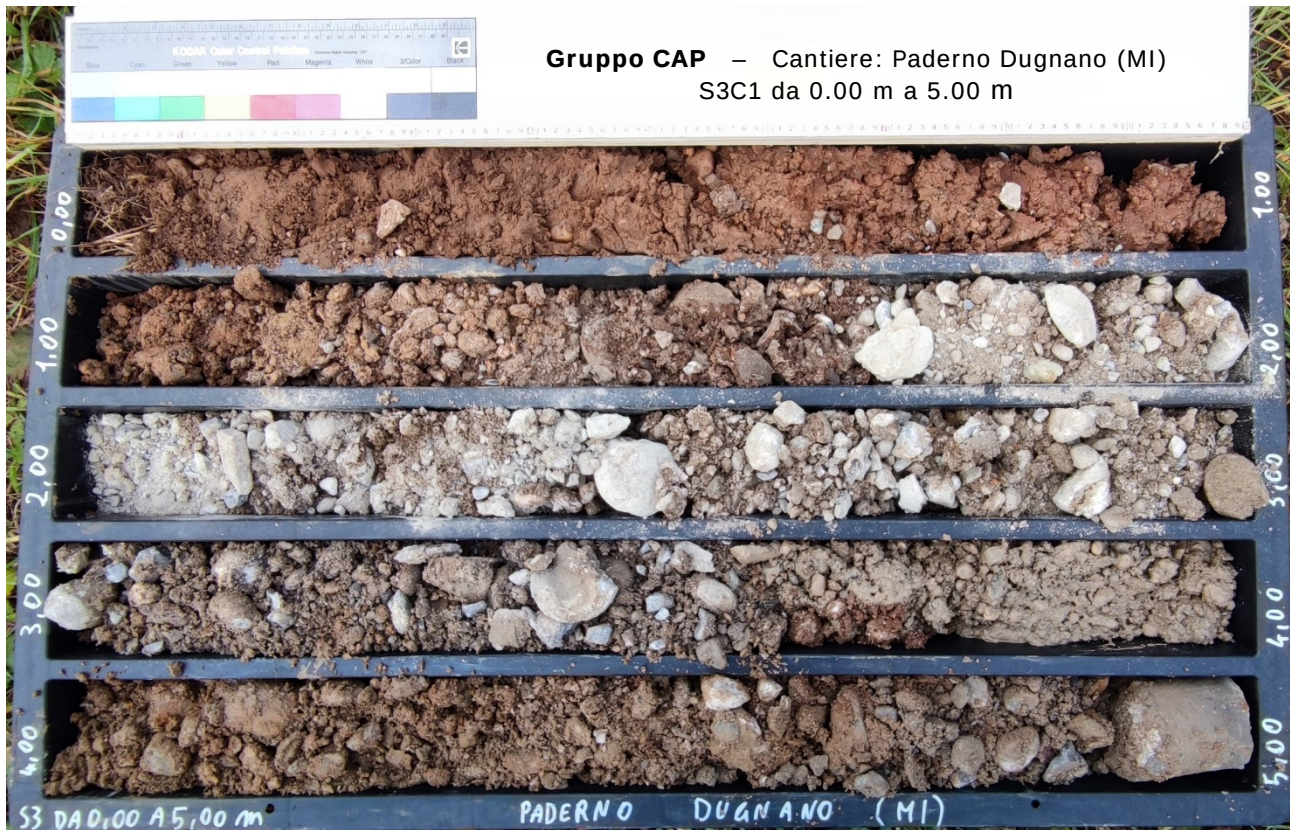
Foto 5. Sondaggio S3 da 0.00 m a 5.00 m.
