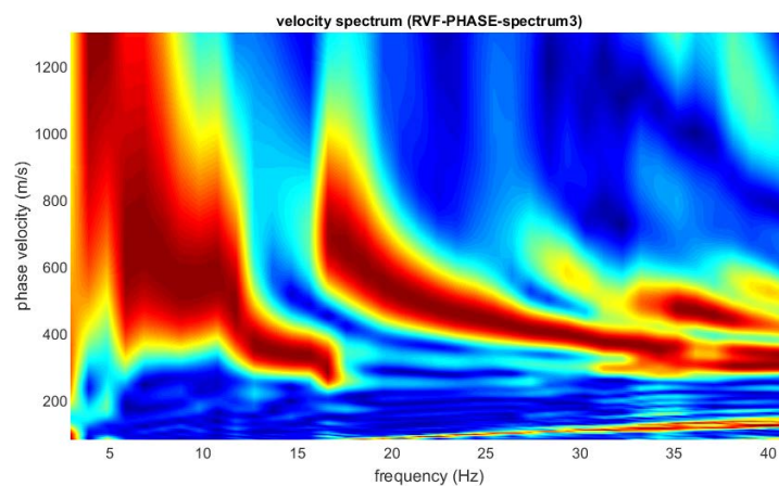
Figura 36. Spettro di velocità, Dataset Onde Rayleigh componente radiale (RVF)
