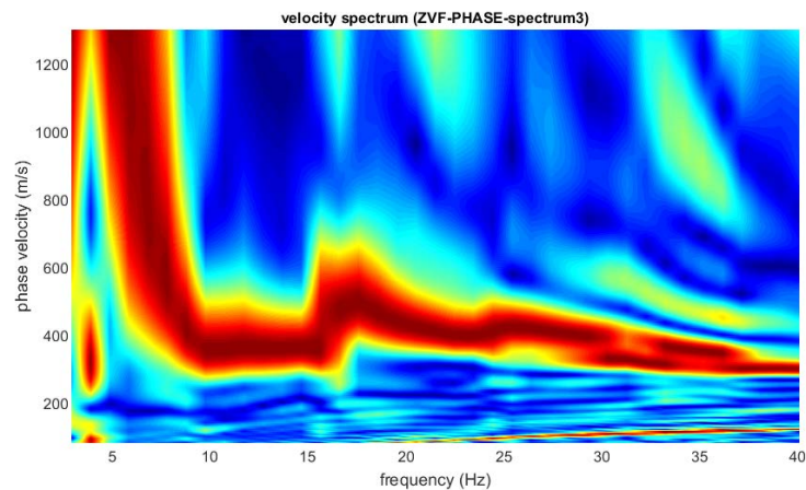
Figura 35. Spettro di velocità, Dataset Onde Rayleigh componente verticale (ZVF)
