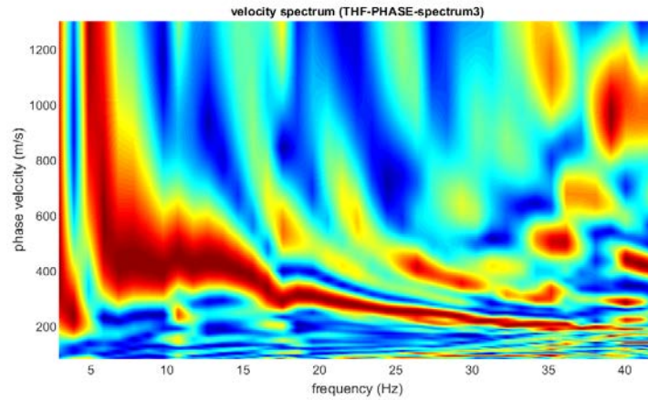
Figura 37. Spettro di velocità, Dataset Onde Love componente orizzontale (THF)
