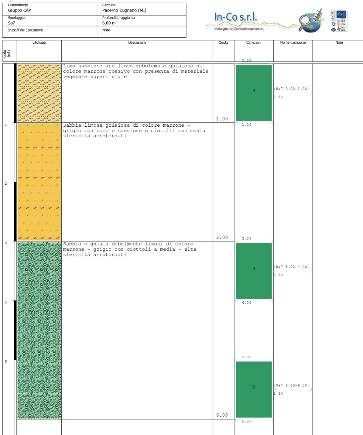
Figura 19. Stratigrafia del sondaggio Sa7.
