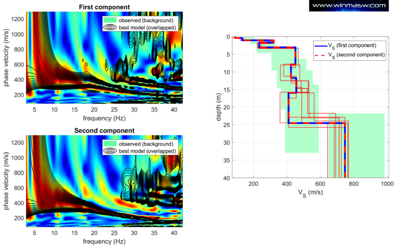
Figura 38. Inversione congiunta delle onde Rayleigh e Love
