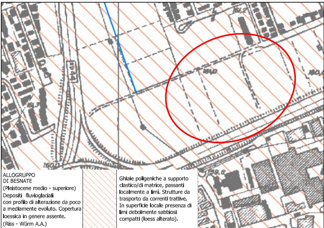
Figura 4. Carta geologica, scala 1:5000, del Comune di Paderno Dugnano
