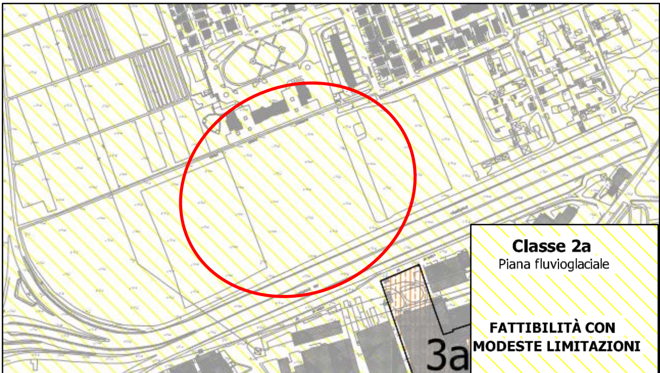
Figura 1. Carta di fattibilità geologica, scala 1:5000, Comune di Paderno Dugnano
