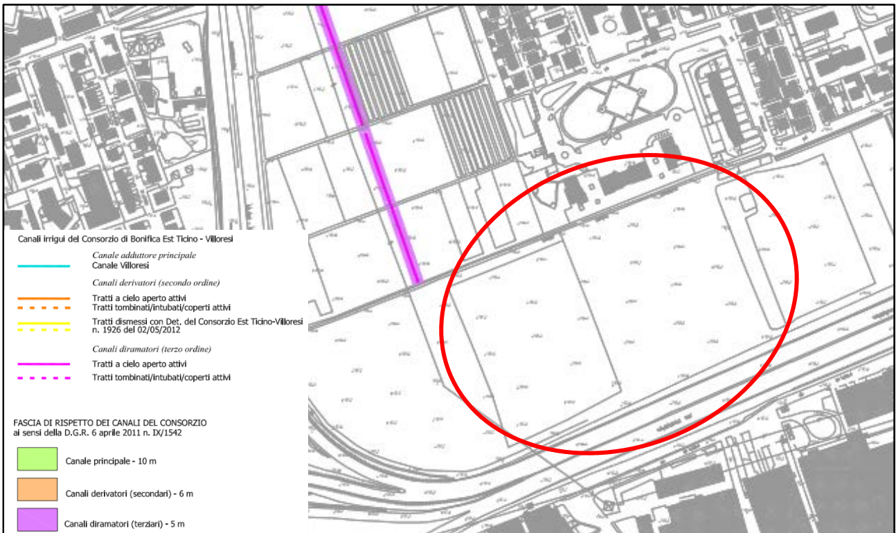
Figura 3. Carta dei Vincoli, scala 1:5000, del Comune di Paderno Dugnano
