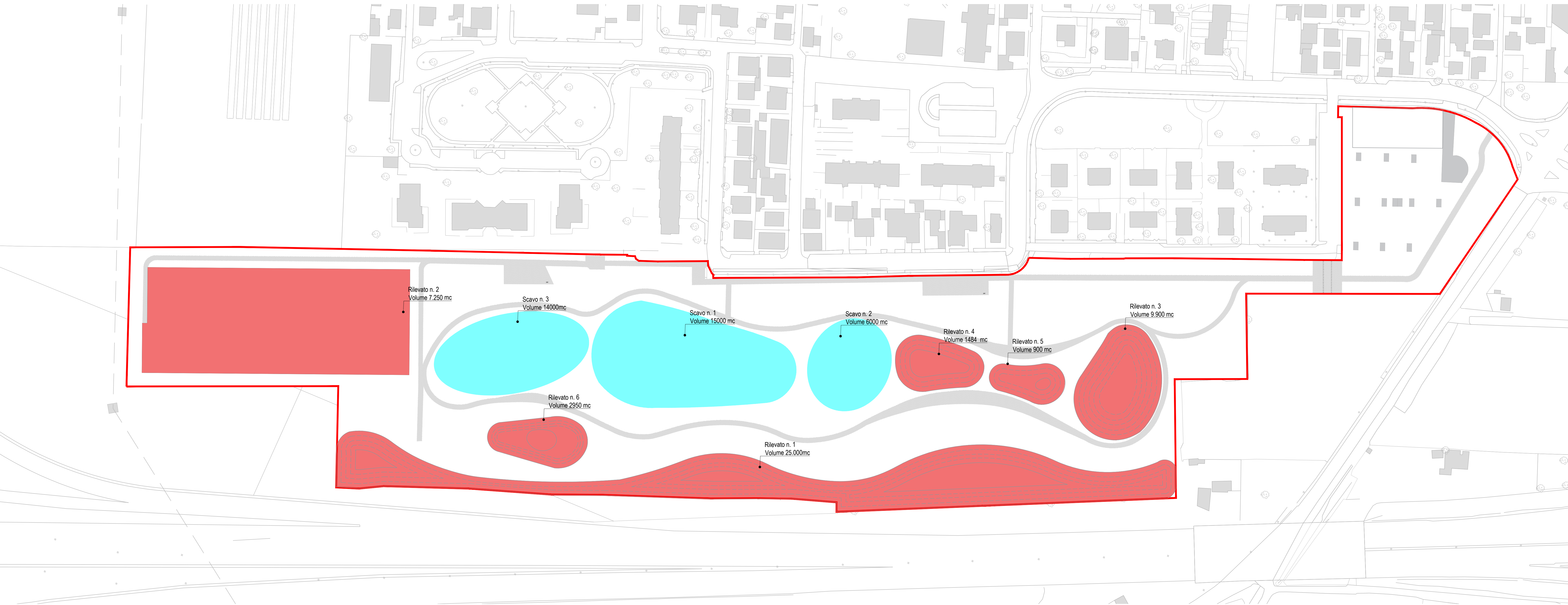
02 PLANIMETRIA SCAVI E RILIEVI DI PROGETTO 1:1000
