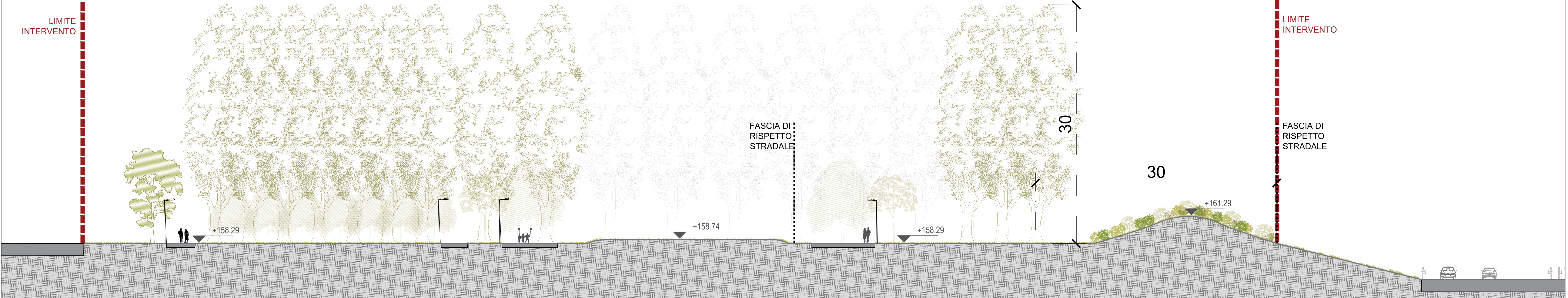
04 SEZIONE IV' 1:200
