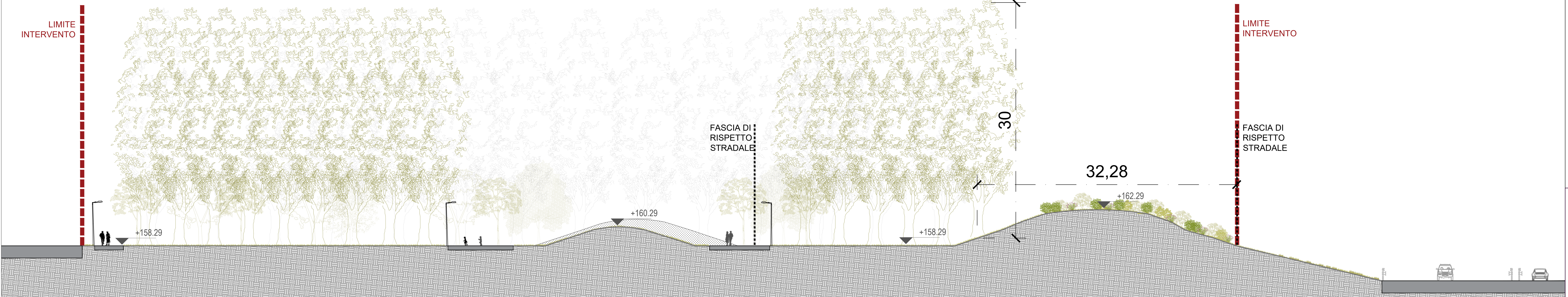
03 SEZIONE III' 1:200
