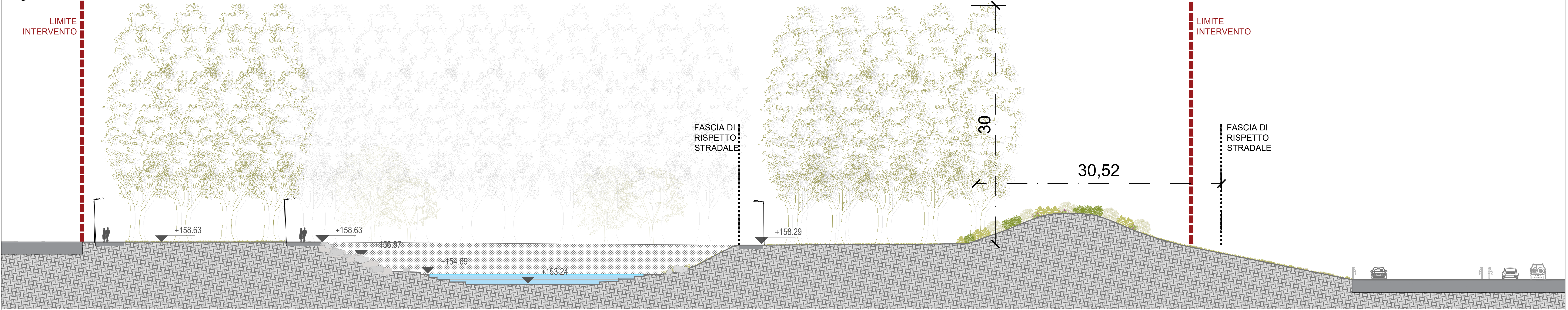
02 SEZIONE II' 1:200
