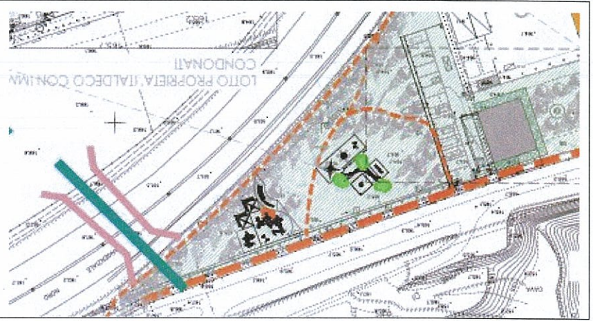
Figura 6 – Estratto dal progetto dell'area in territorio di Cinisello Balsamo destinata a piazzola giochi
